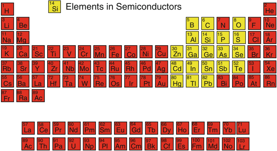
Fig. 4.7 Periodic table
