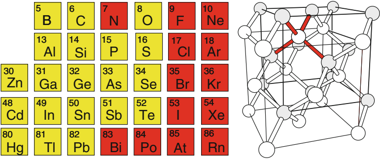
Fig. 4.8 Silicon crystal
