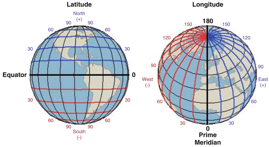
Fig. 4.4 Longitude and latitude
