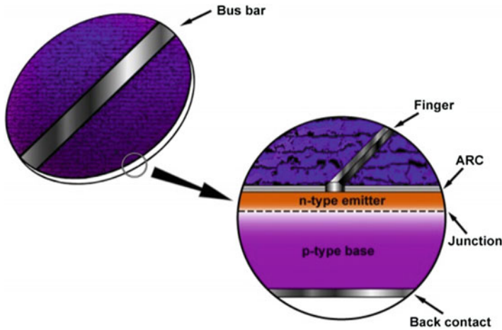
Fig. 4.18 Solar cell
